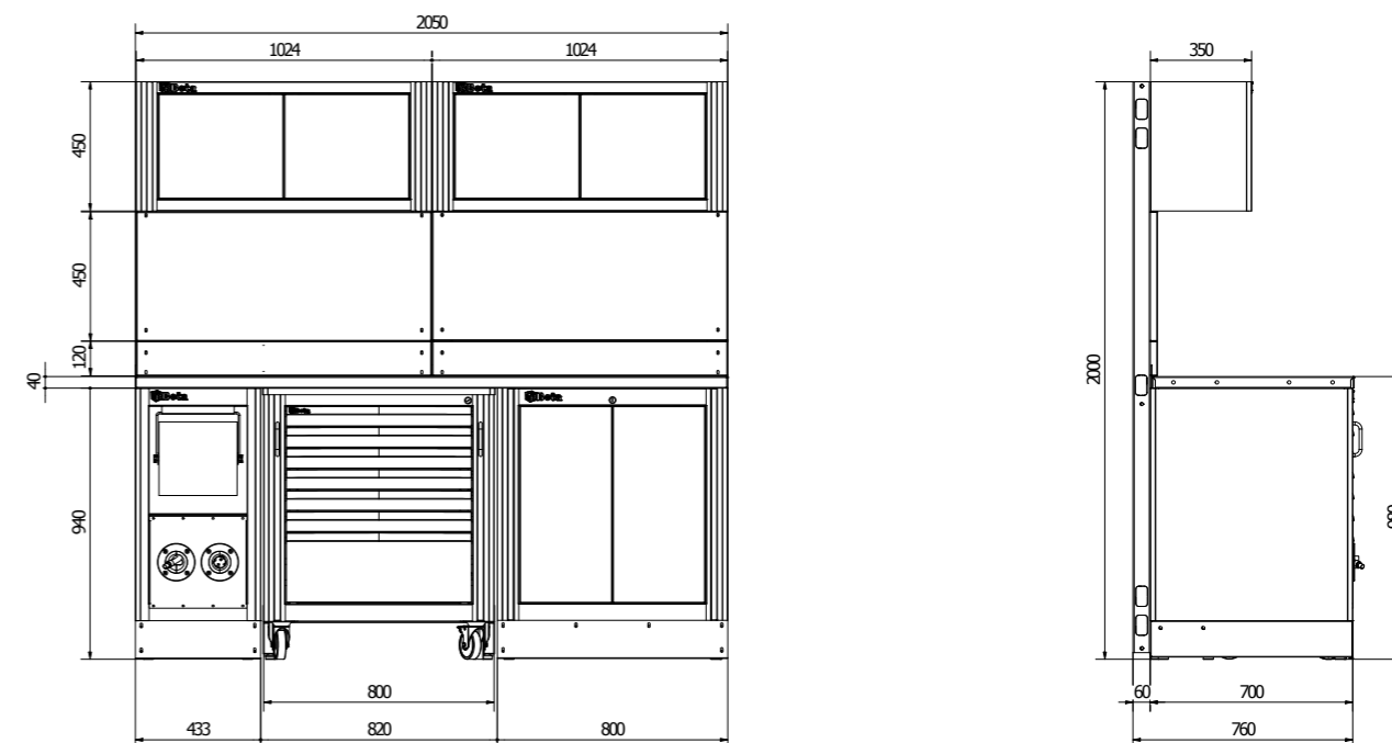
CONFIGURAZIONE 2050 CON PENSILI A DUE ANTE CONFIGURATION 2050 WITH TWO-DOOR WALL CABINETS COD. 3DP99W12IFU
