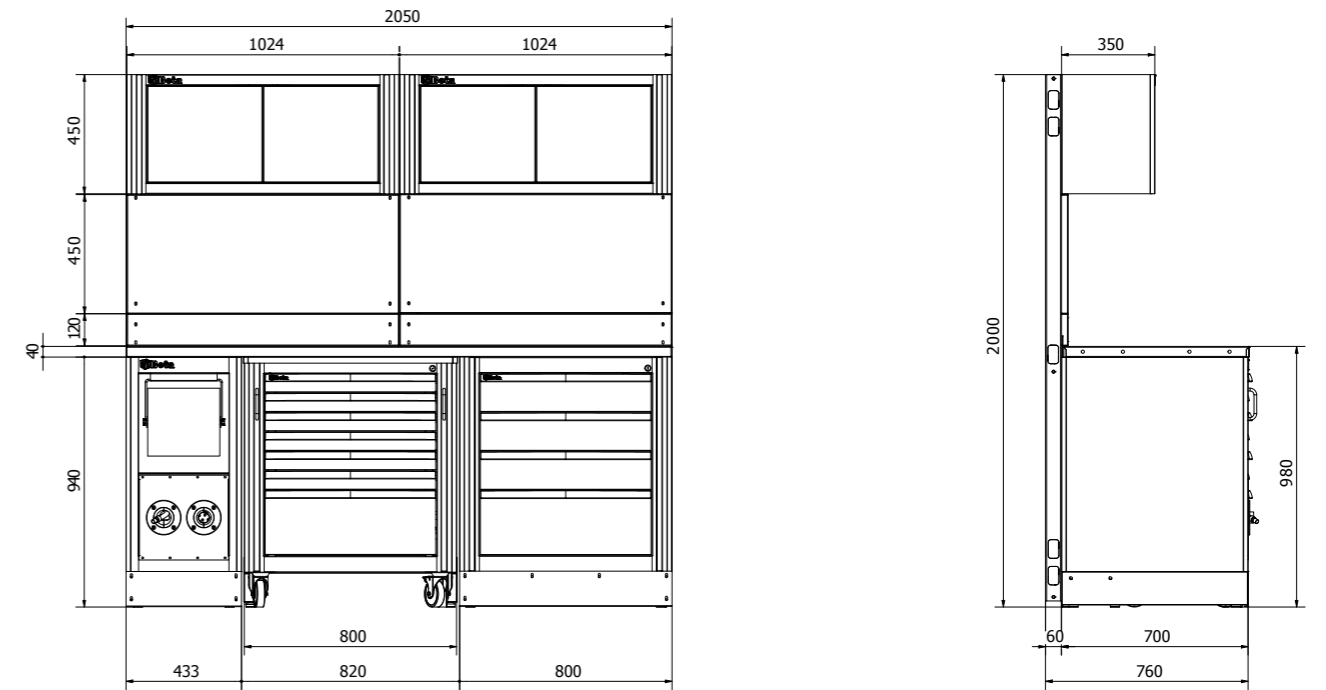
CONFIGURAZIONE 2050 CON PENSILI A DUE ANTE CONFIGURATION 2050 WITH TWO-DOOR WALL CABINETS COD. 3DP99W09IFU
