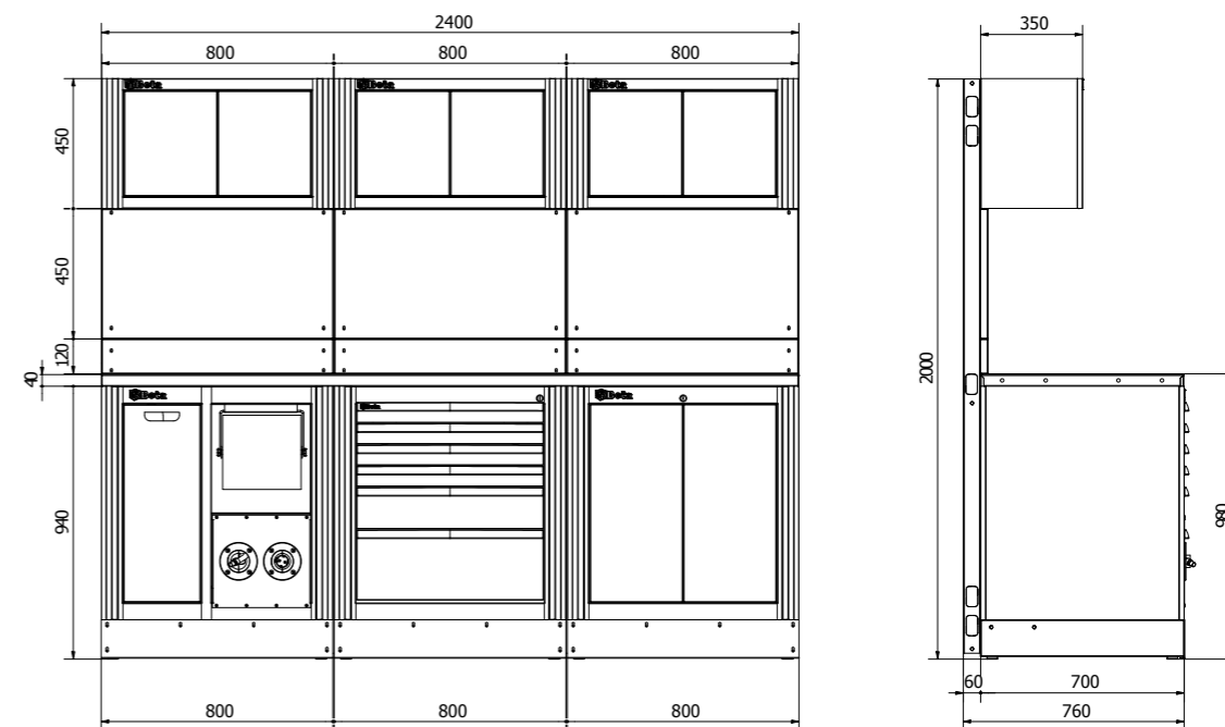
CONFIGURAZIONE 2400 CON PENSILI A DUE ANTE CONFIGURATION 2400 WITH TWO-DOOR WALL CABINETS COD. 3DP99W15IFV
