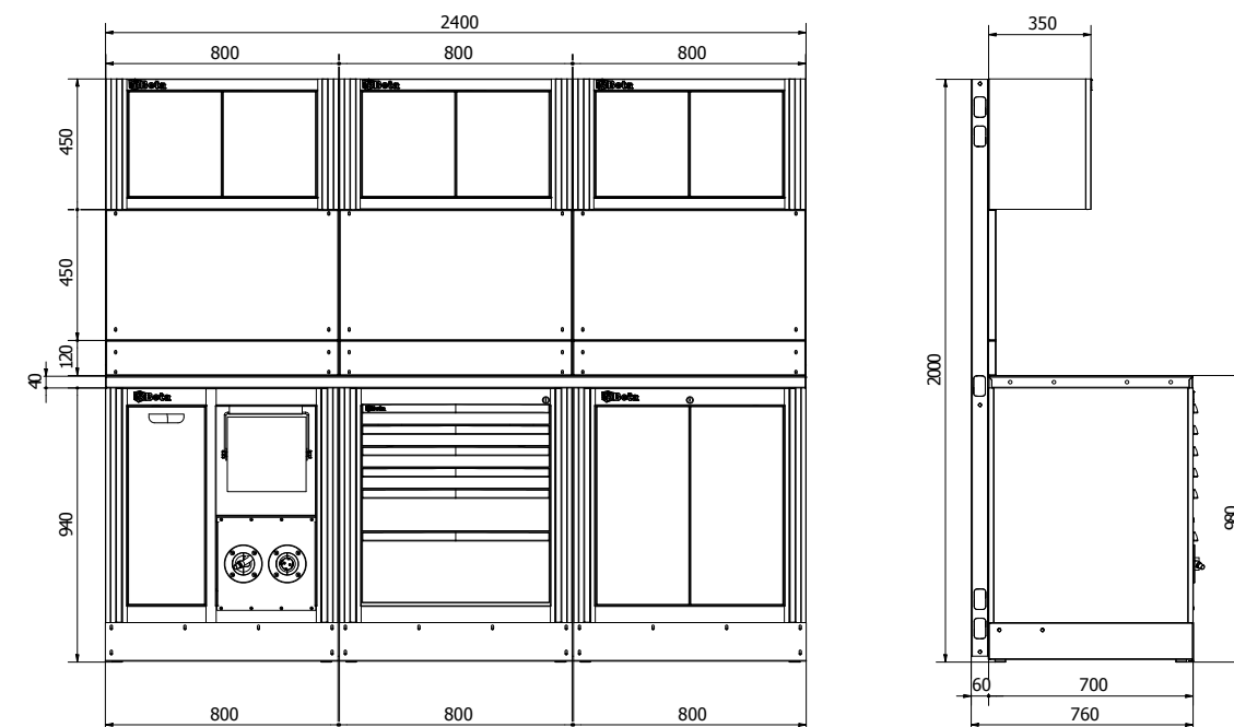
CONFIGURAZIONE 2400 CON PENSILI A DUE ANTE CONFIGURATION 2400 WITH TWO-DOOR WALL CABINETS COD. 3DP99W15IFV
