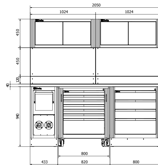
CONFIGURAZIONE 2050 CON PENSILI A DUE ANTE CONFIGURATION 2050 WITH TWO-DOOR WALL CABINETS COD. 3DP99W09IFU
