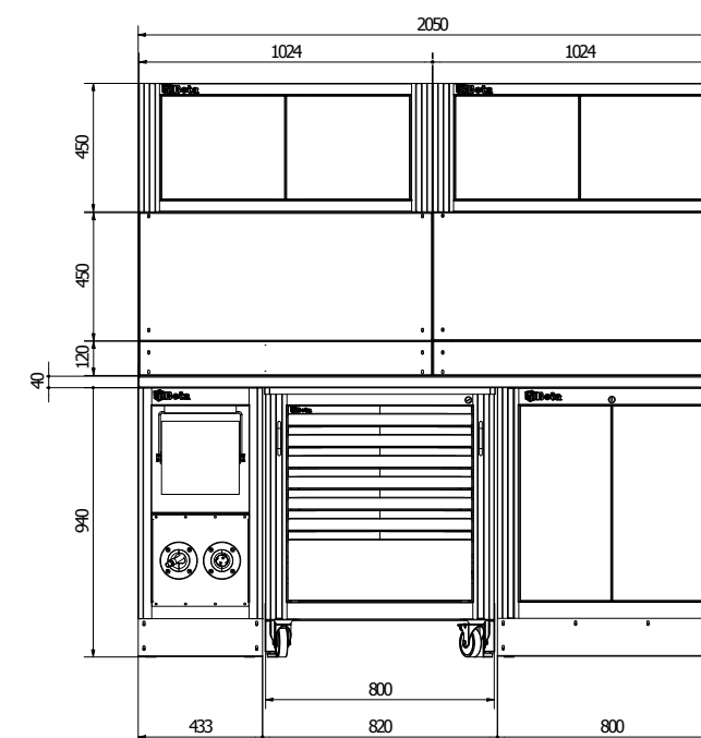
CONFIGURAZIONE 2050 CON PENSILI A DUE ANTE CONFIGURATION 2050 WITH TWO-DOOR WALL CABINETS COD. 3DP99W12IFU
